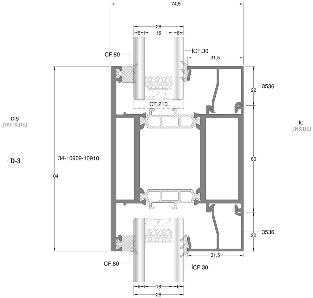
HEMYÜZ DIŞA AÇILIR KAPI DETAY
