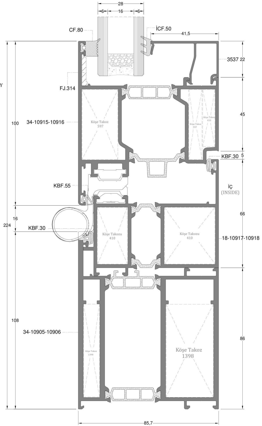
HEMYÜZ DIŞA AÇILIR KAPI DETAY
